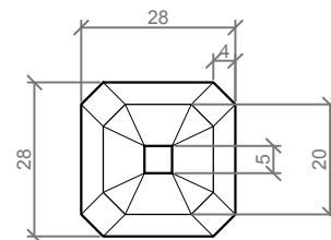
PLANTA / TOP VIEW
