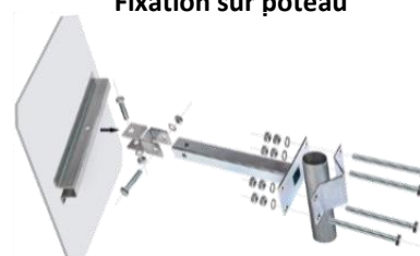
Fixation sur poteau
