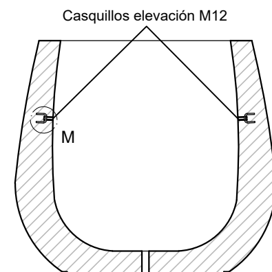
SECCIÓN A-A' / SECTION A-A'
