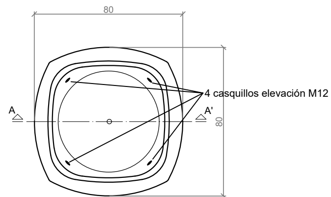
PLANTA / TOP VIEW
